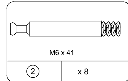
CAM BOLT Perno de la leva BOULON DE CAME TJH2001
