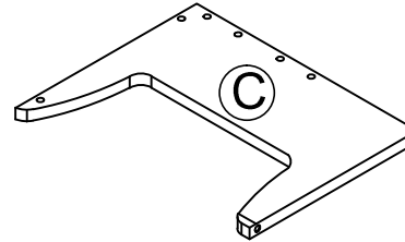
LEFT PANEL Panel izquierdo PANNEAU GAUCHE T9800296033JH
